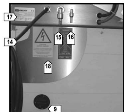
Вид сзади 2-камерных машин серии POLAR
